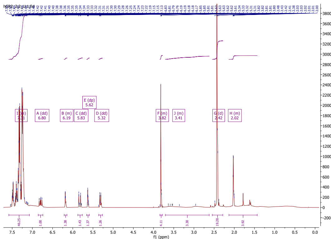
Abb. 16: NMR-Spektrum der Polystyrol- co -Polymethylmethacrylatprobe vor der Fällung.
